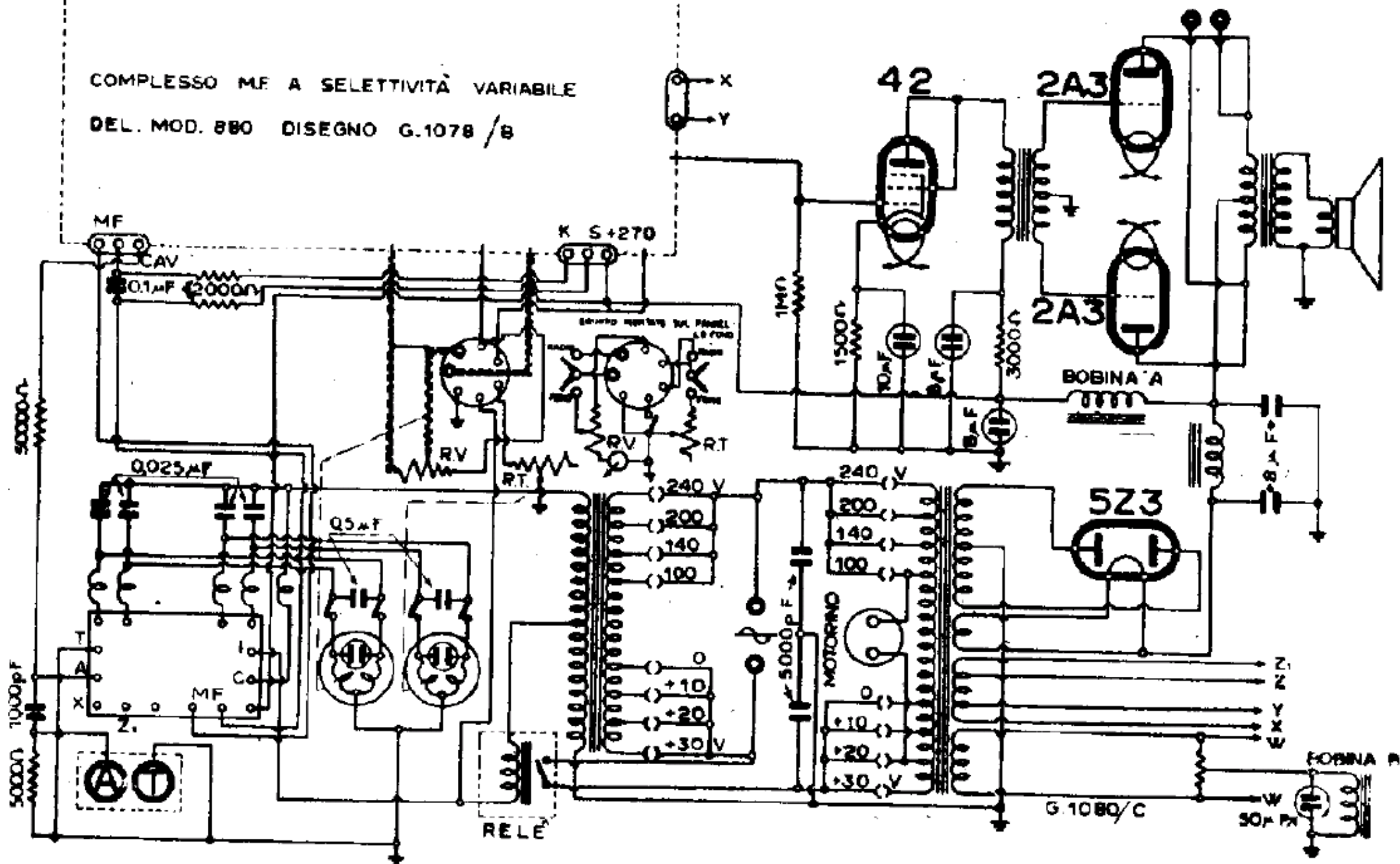
F.I.M.I. - MOD. PHONOLA « 910 » - PARTE BF
